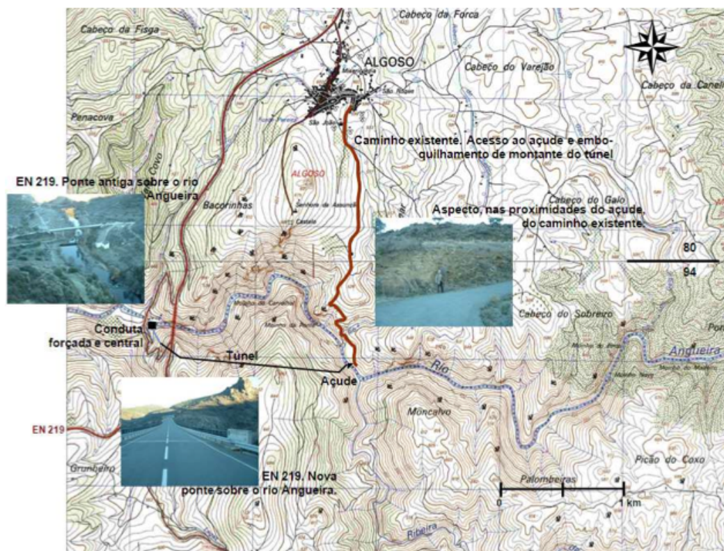
Fig. 4 - Representação dos acessos projectados no âmbito da implementação do o Aproveitamento Hidroelétrico de Algozo – Senhora da Assunção, na margem direita do rio Angueira (extracto da CMP - Escala 1/25 000 (folhas n.º 80 e 94) ( in Estudo de viabilidade técnico-económica do AHE de Algozo - Senhora da Assunção, Hidroerg, Projectos Energéticos- 2014).
