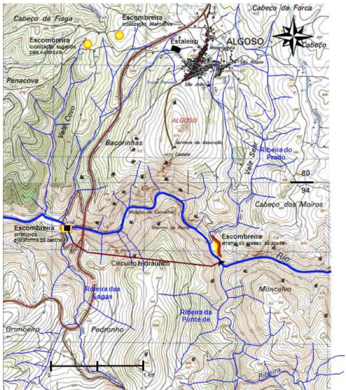
Fig. 6 – Localização das escombreira e estaleiro projectados no âmbito da implementação do o Aproveitamento Hidroeléctrico de Algosó – Senhora da Assunção (extracto da CMP - Escala 1/25 000 (folhas n.º 80 e 94) (in Estudo de viabilidade técnico-económica do AHE de Algosó - Senhora da Assunção, Hidroerg, Projectos Energéticos- 2014).
