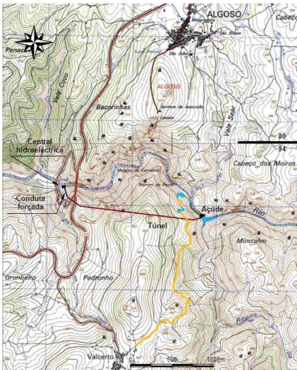
Fig. 5 - Representação do acesso projectado no âmbito da implementação do o Aproveitamento Hidroeléctrico de Algosó – Senhora da Assunção, na margem esquerda do rio Angueira. A amarelo, caminho existente, a azul, trechos a rectificar, a verde prolongamento a executar (extracto da CMP - Escala 1/25 000 (folhas n.º 80 e 94) (in Estudo de viabilidade técnico-económica do AHE de Algosó - Senhora da Assunção, Hidroerg, Projectos Energéticos- 2014).
