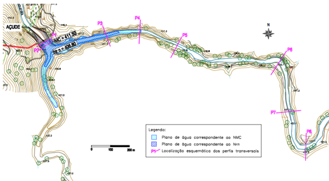
Fig. 2 - Planta geral da albufeira ( in Estudo de viabilidade técnico-económica do AHE de Algosó - Sra da Assunção, Hidroerg, Projectos Energéticos- 2014).
