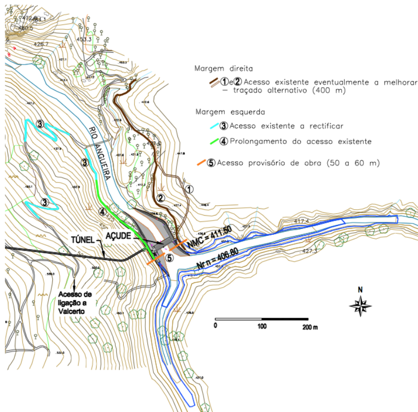
Fig. 15 – Acessos rodoviários que se prevêem utilizar a área envolvente ao açude e emboquilhamento montante do túnel (sobre base cartográfica à escala 1/5000) (in Estudo de viabilidade técnico-económica do AHE de Algosó - Senhora da Assunção, Hidroerg, Projectos Energéticos- 2014).
