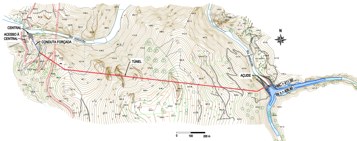
Fig. 1 - Representação esquemática do circuito hidráulico projectado para o Aproveitamento Hidroeléctrico de Algos – Sra. da Assunção. A. Implantação cartográfica na CMP - Escala 1/25 000 (folhas n.º 80 e 94); B. Planta geral do circuito hidráulico. ( in Estudo de viabilidade técnico-económica do AHE de Algos - Sra da Assunção, Hidroerg, Projectos Energéticos- 2014).
